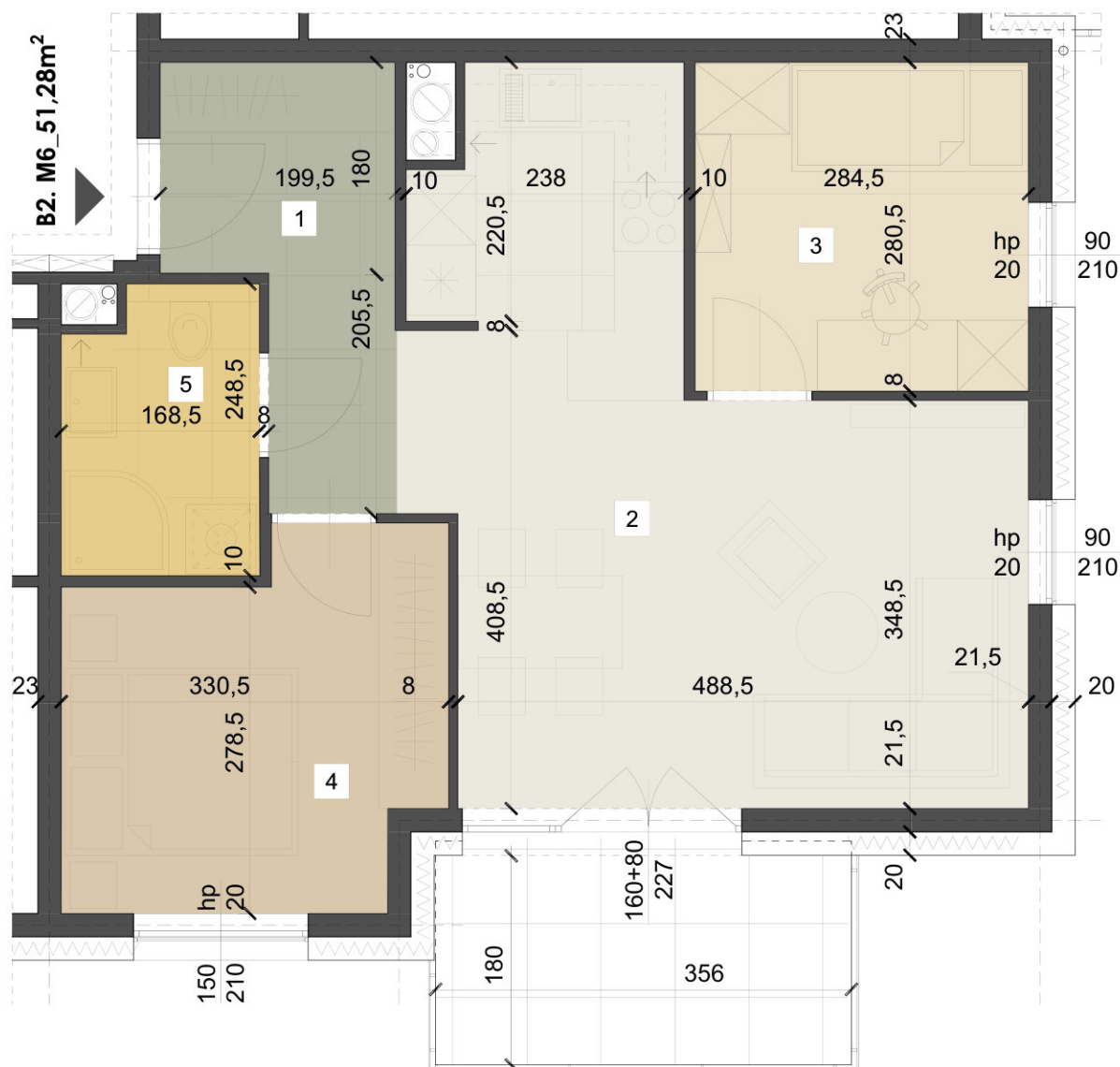
MIESZKANIE B2. M6
