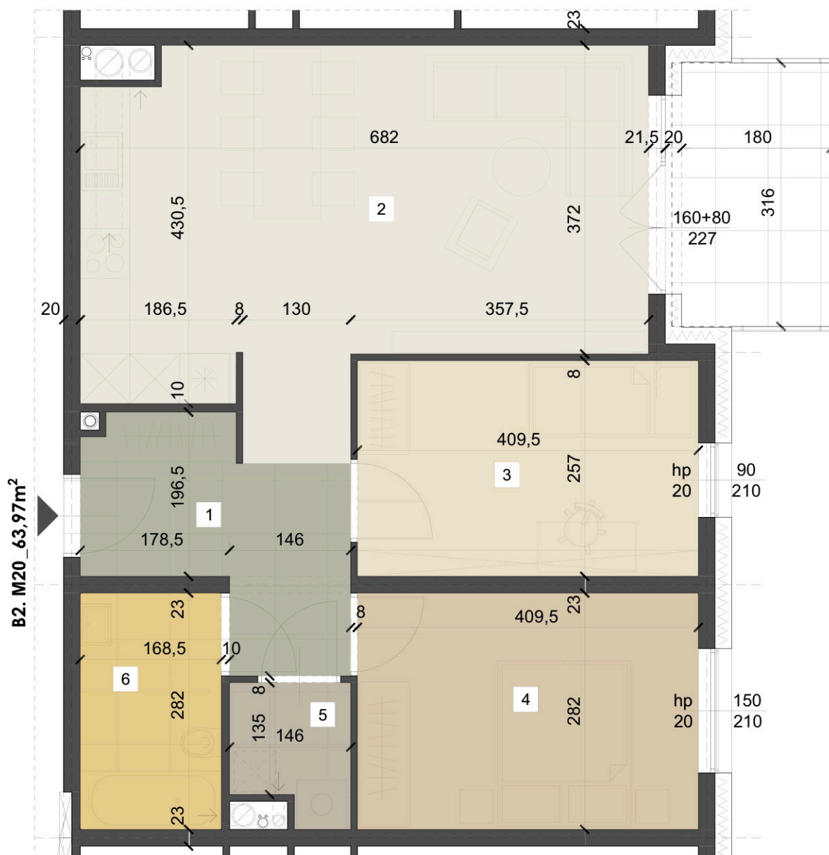
MIESZKANIE _ B2. M20
