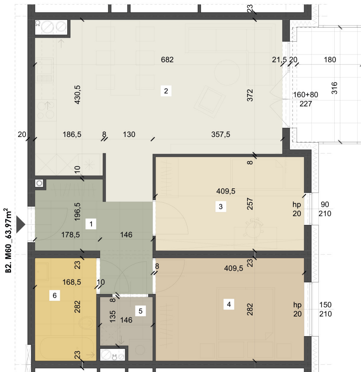
MIESZKANIE _ B2. M60
